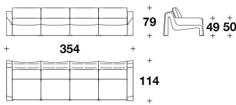
ING (D4) DIVANO 4 POSTI / 4 SEATER SOFA 354x114x79H. - H.S.49cm 139 1/2x45x31H. - H.S.19 1/4"
