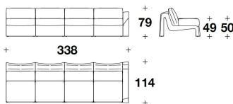
ING (E4D) - ING (E4S) ELEMENTO 4 POSTI CON BRACCIOLO DX O SX / 4 SEATER ELEMENT WITH RIGHT OR LEFT ARMREST 338x114x79H. - H.S.49cm 133x45x31H. - H.S.19 1/4"
