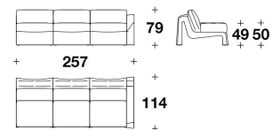
ING (E3D) - ING (E3S) ELEMENTO 3 POSTI CON BRACCIOLO DX O SX / 3 SEATER ELEMENT WITH RIGHT OR LEFT ARMREST 257x114x79H. - H.S.49cm 101 1/3x45x31H. - H.S.19 1/4"
